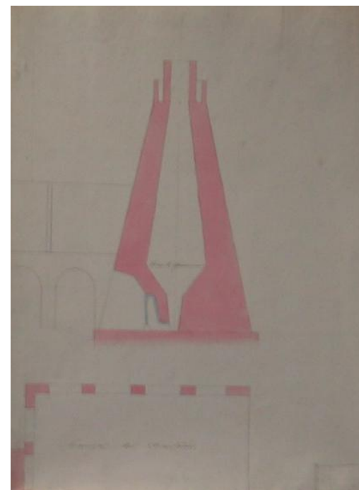
Plan des Haut-Fourneaux, Denain (1834)
